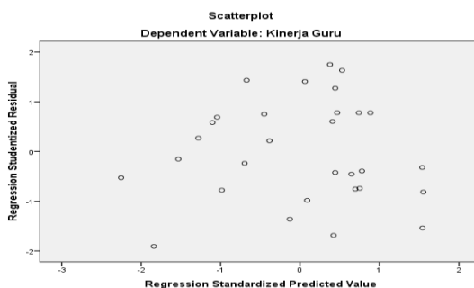
Gambar 5. Uji Heterokedastisitas
