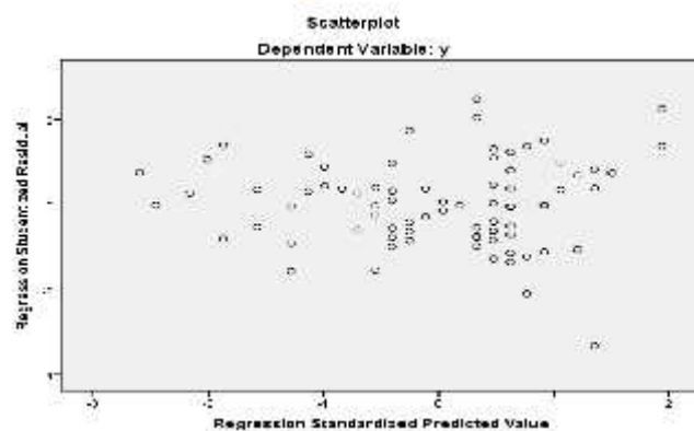
Gambar 1.4 Uji Heteroskedastisitas
