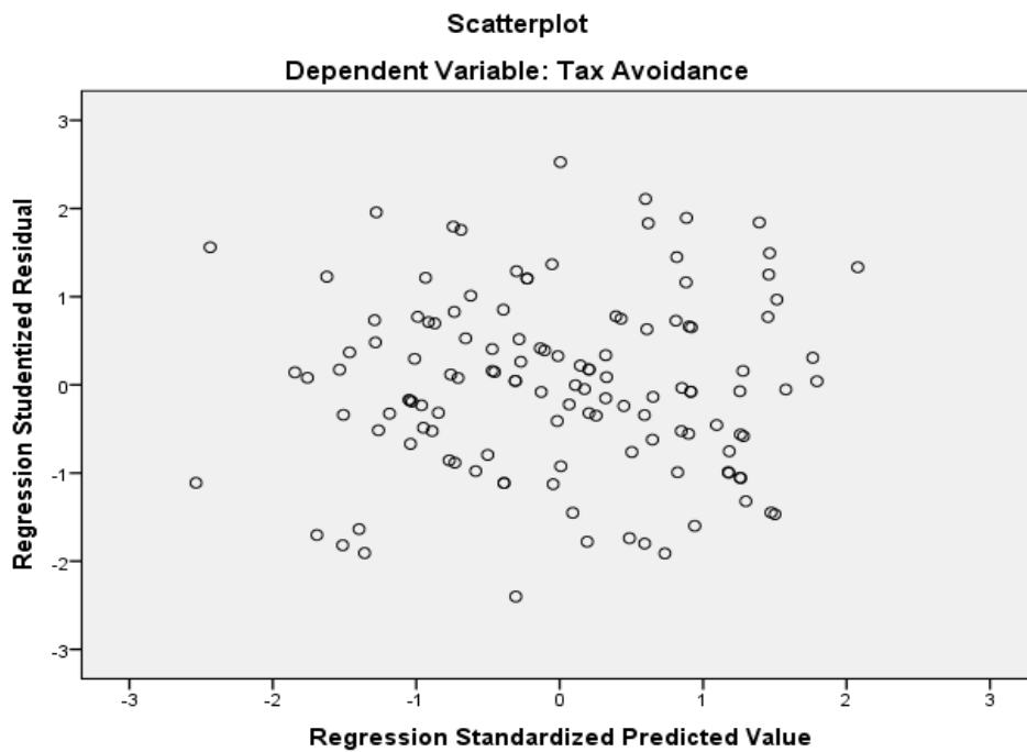
Gambar 3.3 Uji Heteroskedastisitas
