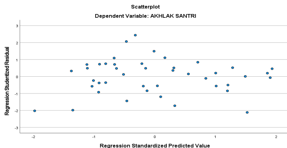
Gambar 4.1 Uji Heteroskedastisitas
